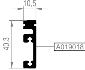
Ölçek / Scale 1:2
