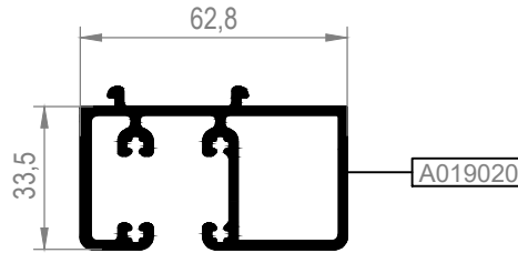
Ölçek / Scale 1:2
