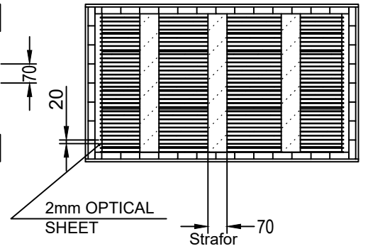
KESİT H
