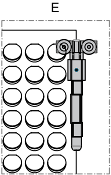
07.31.01 ÜST KAFA ARABA TOP END ROLLER
