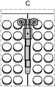
07.31.02 ÜST ORTA ARABA TOP CENTRAL ROLLER
