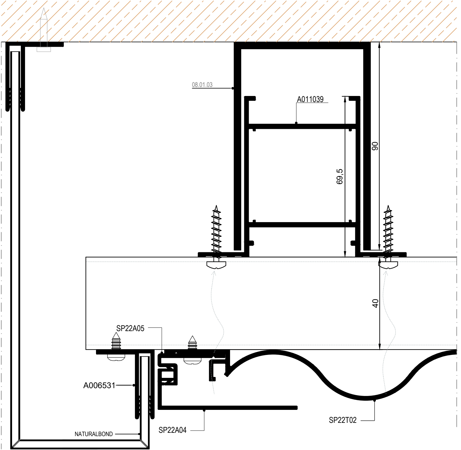
DÜŞEY VERTICAL
