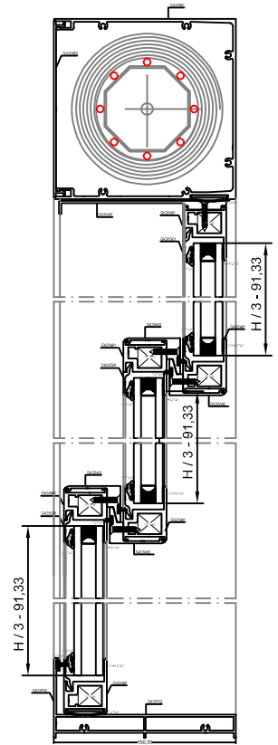
D-D Kesiti
