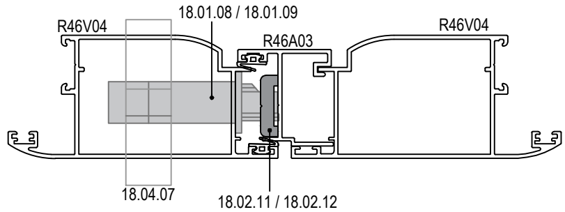
**DIŞA AÇILIM HEMYÜZ ORTA BİRLEŞİM DETAYI İÇİN (R46 A 03) **OUTWARD OPENING FLUSH DOOR ADAPTER DETAIL (R46 A 03)
