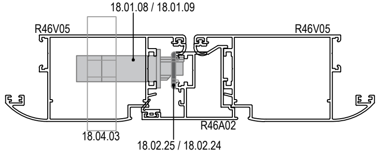
**İÇE AÇILIM BİNİLİ ORTA BİRLEŞİM DETAYI İÇİN **INWARD OPENING DOOR DETAIL
