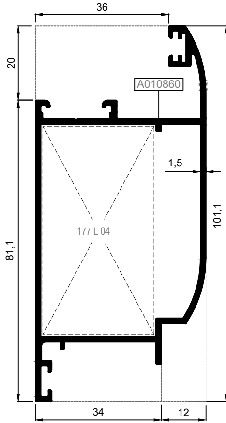
İÇE AÇILIM HEMYÜZ KAPI KANAT PROFİLİ INWARD OPENING FLUSH DOOR VENT PROFILE
